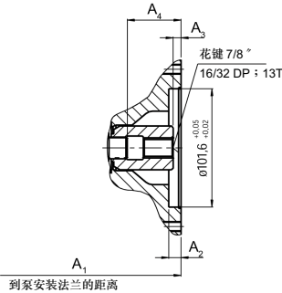
剖面 A - B
