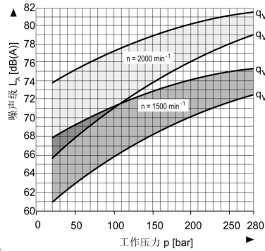
规格 100
