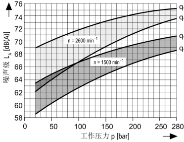
规格 71
