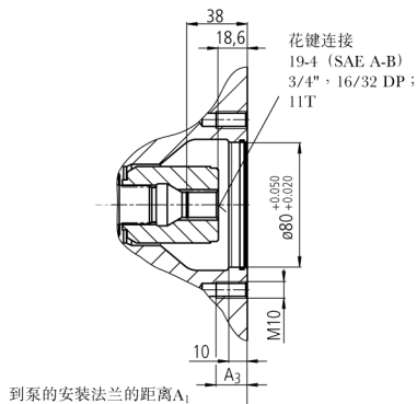
A-B剖面
