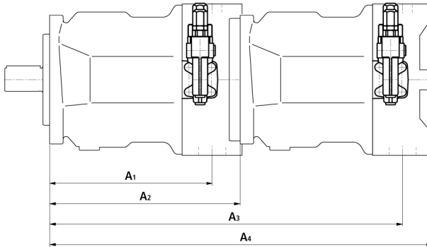
A10VSO + A10VSO
