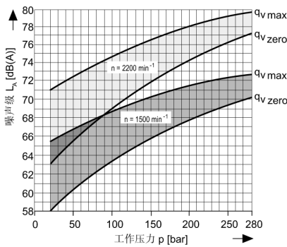
规格 71
