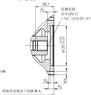
A - B 剖面
