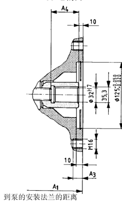
A - B 剖面
