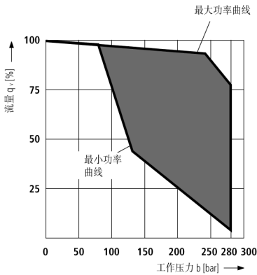
静态工作曲线
