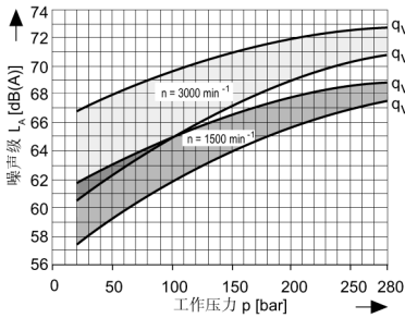
规格 45
