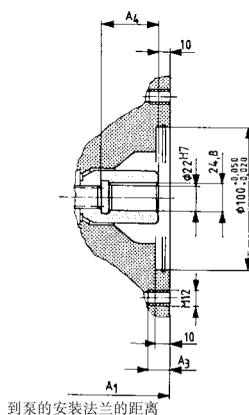
A-B剖面
