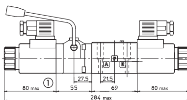
DHE(R)-A-06*/MO DHE(R)-A-07*/MO (虚线)
