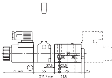
DHE(R)-A-06*/MV DHE(R)-A-07*/MV (虚线) ①=DHE先导阀要短3mm ②=DHE先导阀要短2mm
