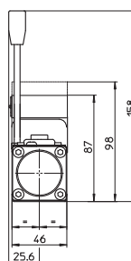
DHA/*-06*/MO DHA/UL-*06*/MV(虚线)
