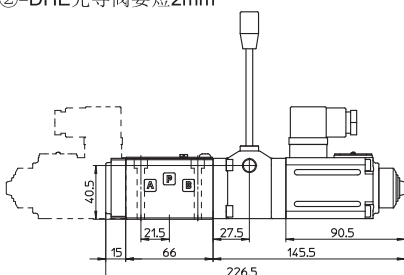
DHZO-A-05*/MV DHZO-A-07*/MV (虚线)
