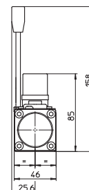
质量: 2.8kg (单电磁铁) 质量: 3.5kg (双电磁铁)
