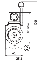
DHE(R)-A-06*/MO DHE(R)-A-07*/MO (虚线)
