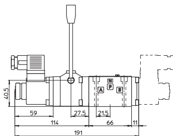
DHI*-06*/MV DHI*-07*/MV(虚线)
